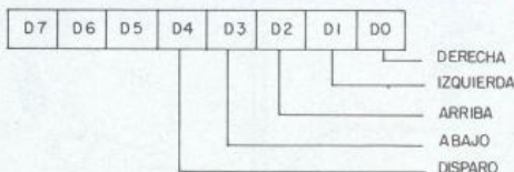
Asignación de los bits del bus de datos a las posiciones de la palanca.
